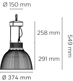
CAMPANA 14/90
